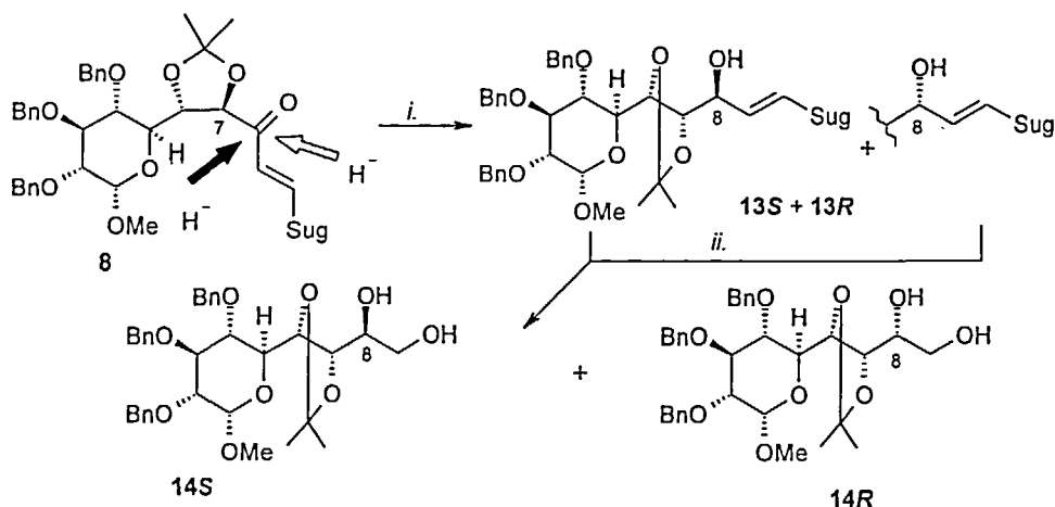
Scheme 3. i. Zn(BH_4)_2 , ether, 0 °C; ii. O_3 , CH_2Cl_2 , -78 °C, then NaBH_4
